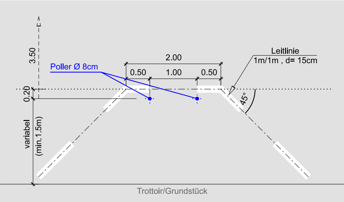
Detail Markierung, 1:10
