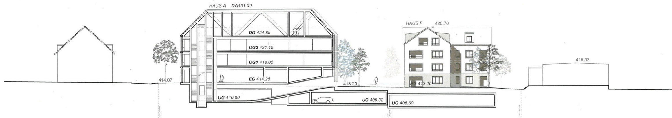
SCHNITT B-B
