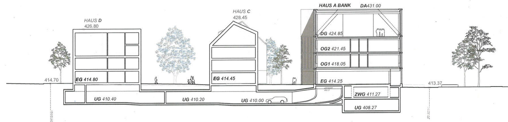
SCHNITT 2-2
